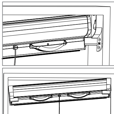
3 Introducir el cajón en el cubre cabezal fijado y luego empujar el otro lado del cajón hacia arriba.
