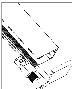
5 Introducir los pies en las guías respetando el sentido de inserción correcto y obteniendo lo que se ve en la segunda imagen arriba.
