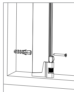
7 Fijar las guías.
