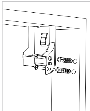
1 Fijar uno de los dos cubre cabezales.
