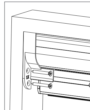
4 Fijar el otro cubre cabezal.
