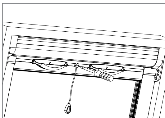
9 Introducir el bloqueo en el perfil barra manilla y girar de 90° utilizando un destornillador plano.
