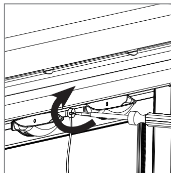
7 Introducir el bloqueo en el perfil barra manilla y girar de 90° utilizando un destornillador plano.
