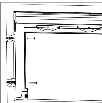
5 Fijar las guías.
