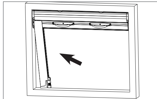
4 Introducir las guías en las embocaduras de los cubre cabezales.
