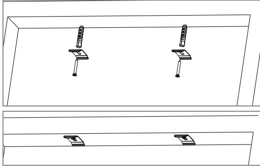
1 Perforar el hueco en correspondencia de los puntos donde se colocarán las clips. Fijar las clips en la jamba.
